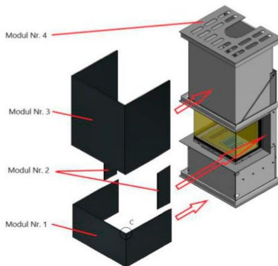
Kaminmodule zur Kaminanlage mit Keramik
